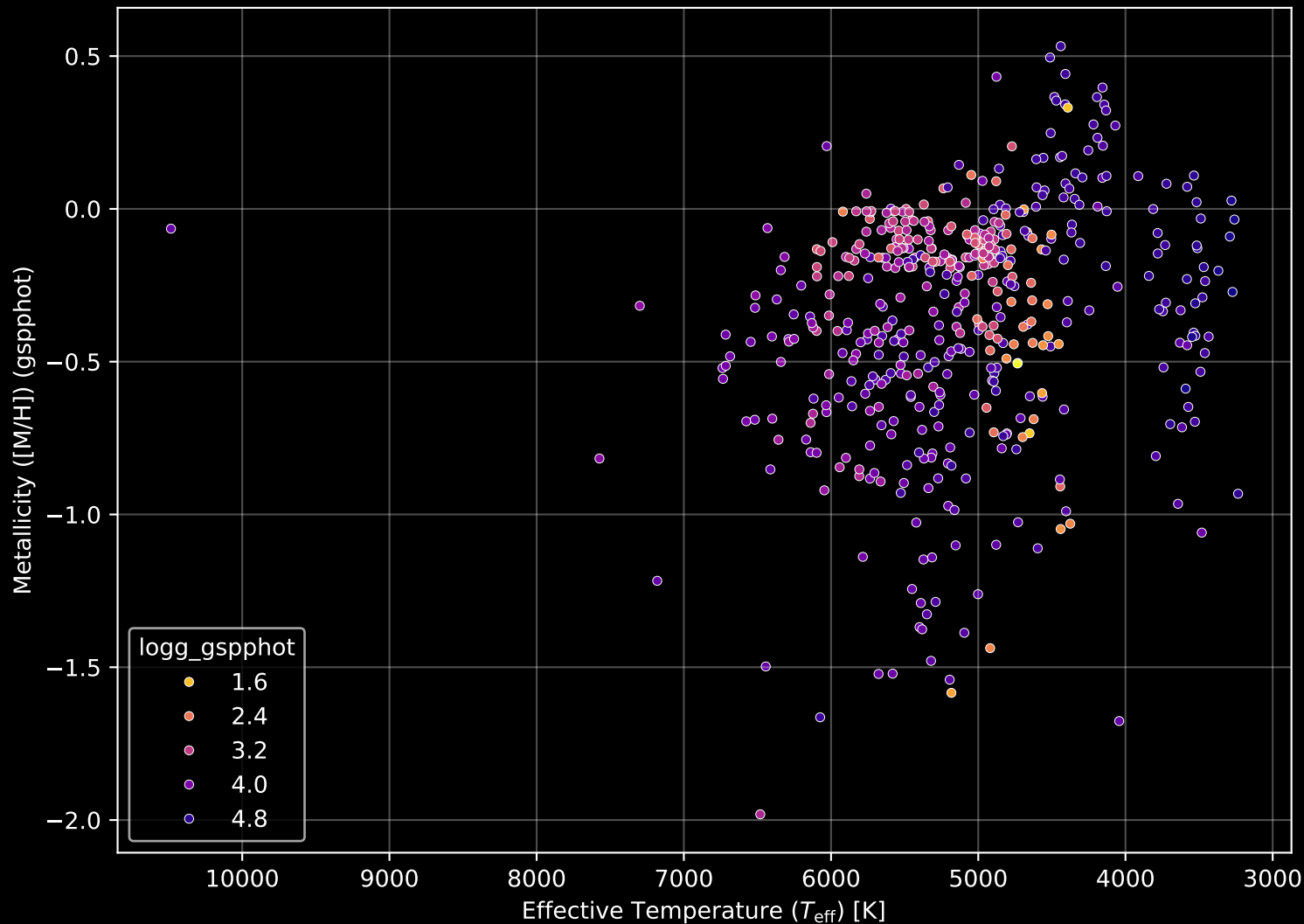
APOGEE DR17 Field: [320+45] Stellar Population Parameters (n= 483)
